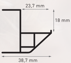
Normaal 30 mm
