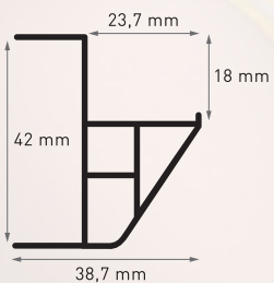
Normaal 40 mm
