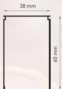
Ondergeleider
